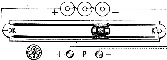
Graphite rheostat.
